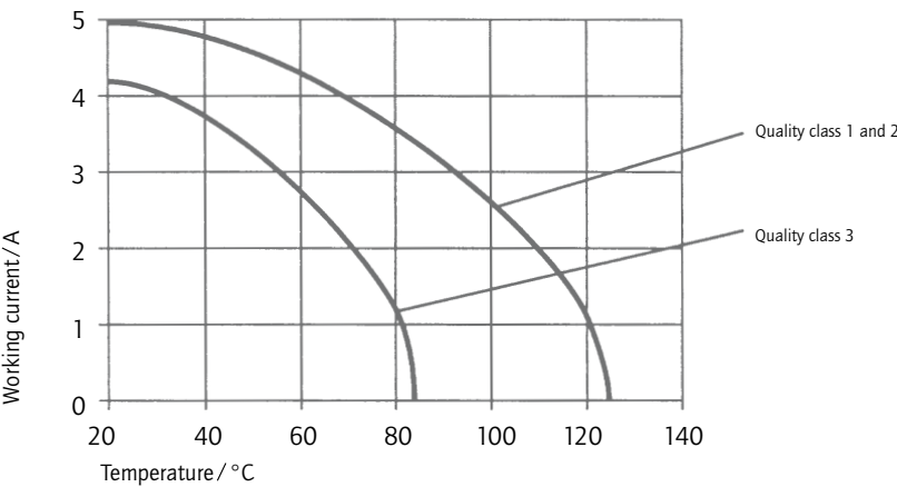
Derating-Diagramm DIN 41617
