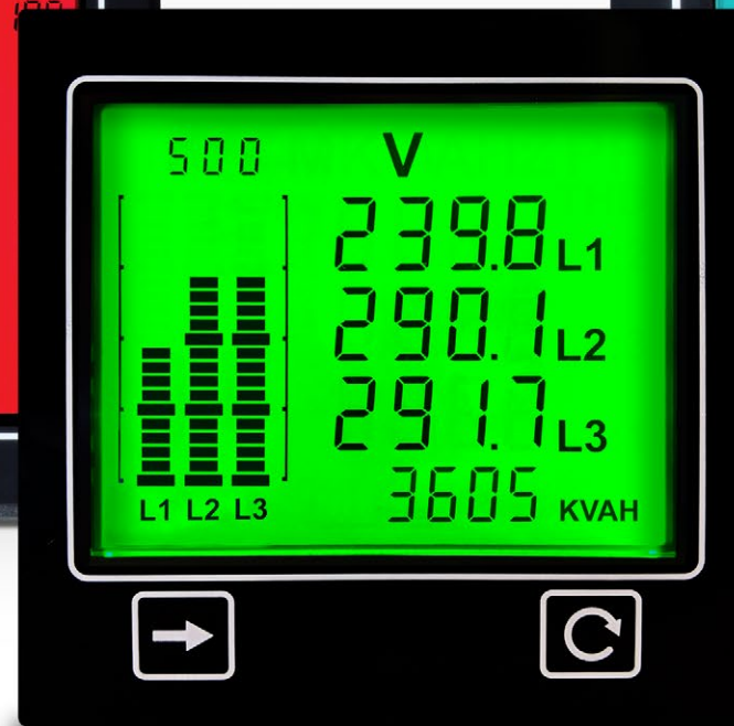
APM Power Meter
